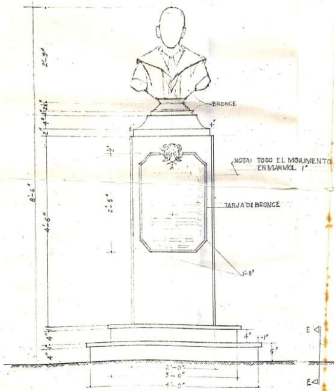
ELEVACION DE LOS 4 LADOS 1/2" = 1'-0"
